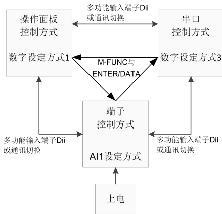
图6-63 三地控制需求（这个图片中的“M-FUNC”更改为“JOG”“ENTER/DATA”更改为“SET”）
