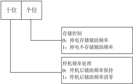
图6-69 数字辅助频率控制设定
