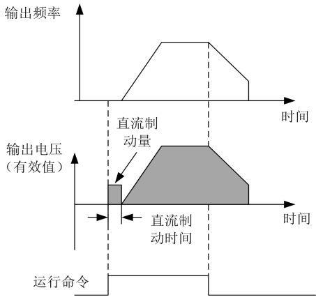
图6-9 起动方式1说明
