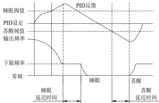
图 6-44 睡眠与苏醒功能示意图
