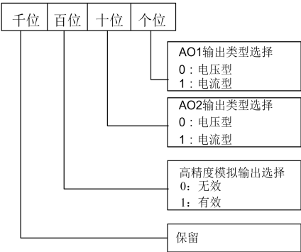
图6-34 模拟输出类型设定
