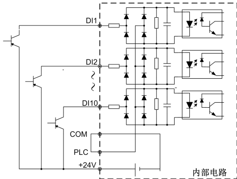
图 3-8 外部电源供电 NPN 图（OC）
