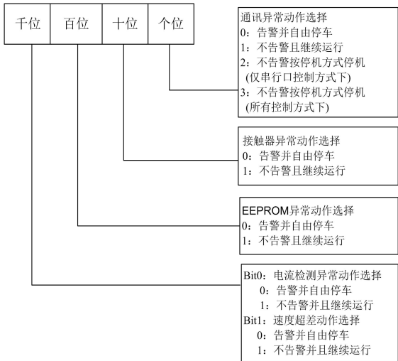
图6-56 保护动作选择1设定
