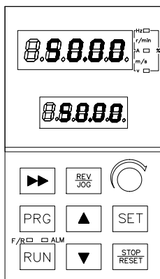
图 4-4 停机参数显示状态
