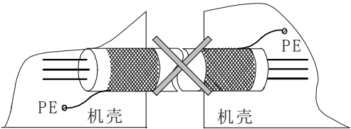
图3-17 错误的屏蔽接地方法
