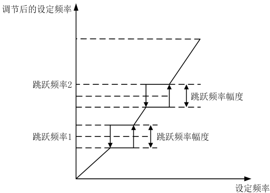
图 6-13 频率跳跃示意图
