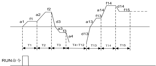
图6-47 PLC单循环后保持方式
