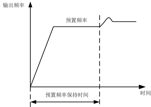
图6-43 闭环预置频率运行示意图
