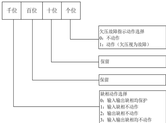
图6-55 保护动作选择2设定
