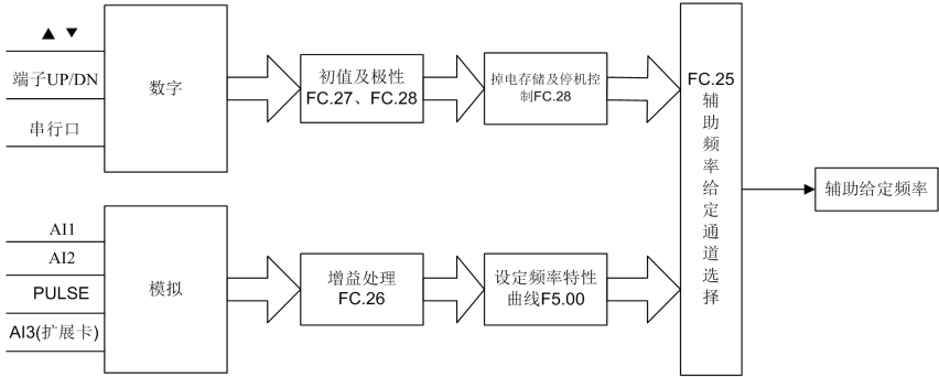
图6-66 辅助频率给定通道示意图
