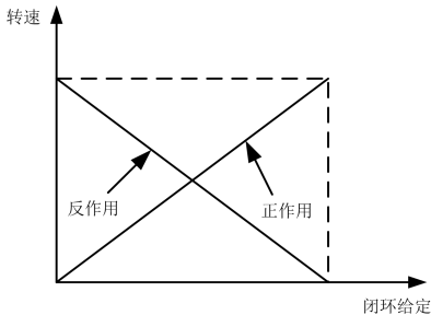
图6-39 闭环调节特性示意图
