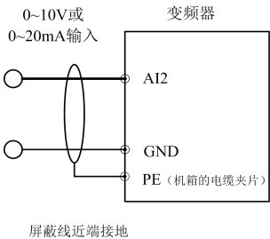
图 3-5 模拟输入端子配线图
