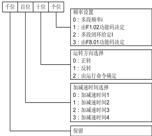
图6-51 PLC阶段 i 设置（ i =1~15）
