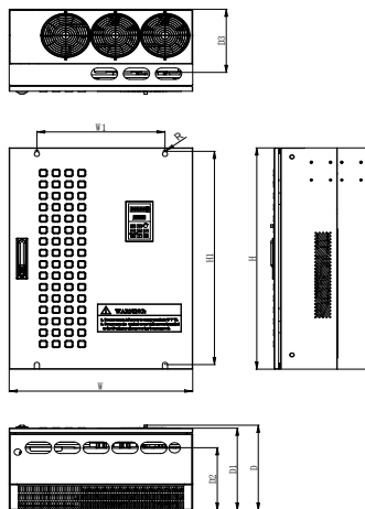
(a) 185KW~200KW 规格尺寸(壁挂)
