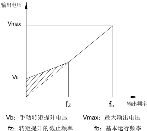
图 6-16 转矩提升示意图
