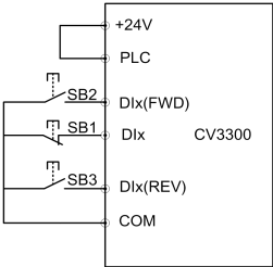
图6-27 三线式运转模式1
