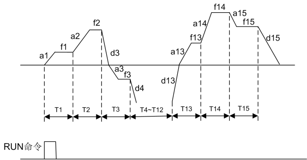
图6-46 PLC单循环后停机方式
