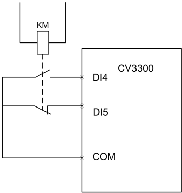
图6-24 外部设备故障常开/常闭输入示意图
