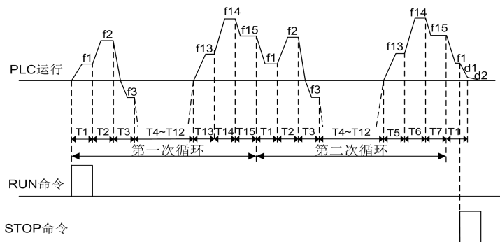
图6-48 PLC连续循环方式
