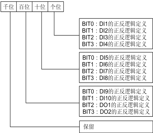
图6-32 端子正反逻辑设定
