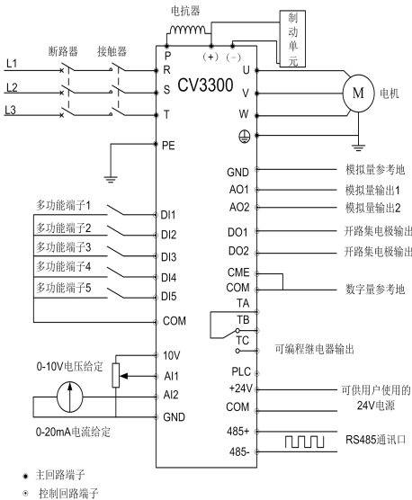
图 3-6 基本运行配线图
