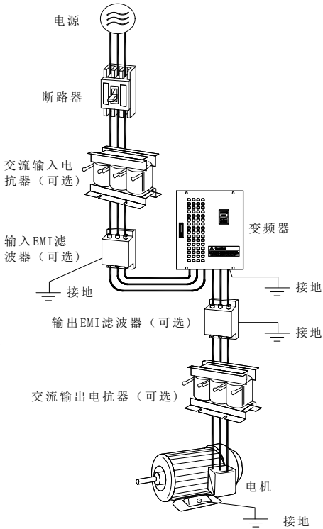
图 3-3 变频器与选配件的连接
