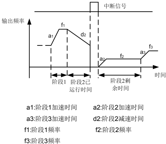
图6-49 PLC起动方式1
