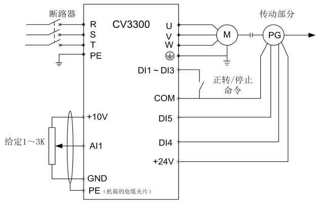
图6-36 PG速度闭环控制系统接线图
