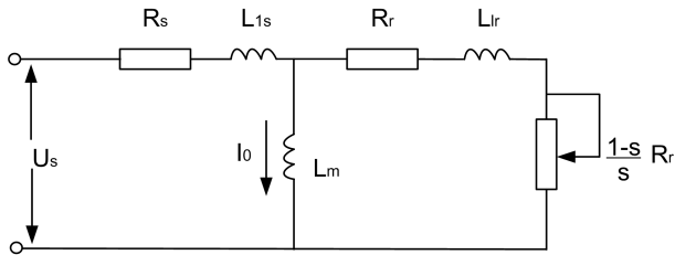
图6-15 异步电机稳态等效电路图
