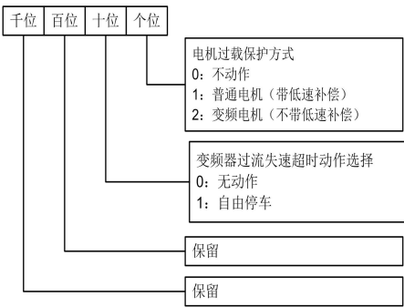
图6-52 保护方式选择设定
