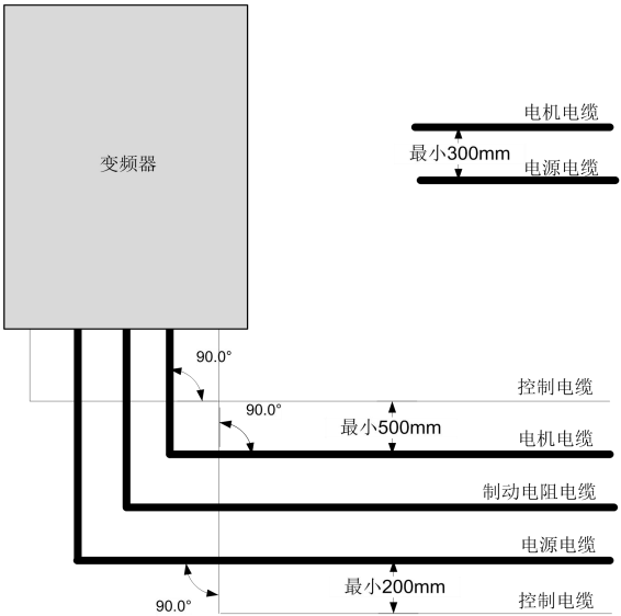
图3-11 系统配线要求
