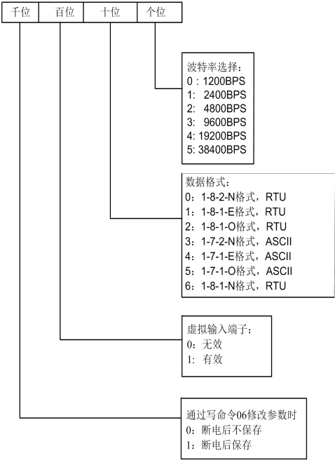
图 6-57 通讯配置设定
