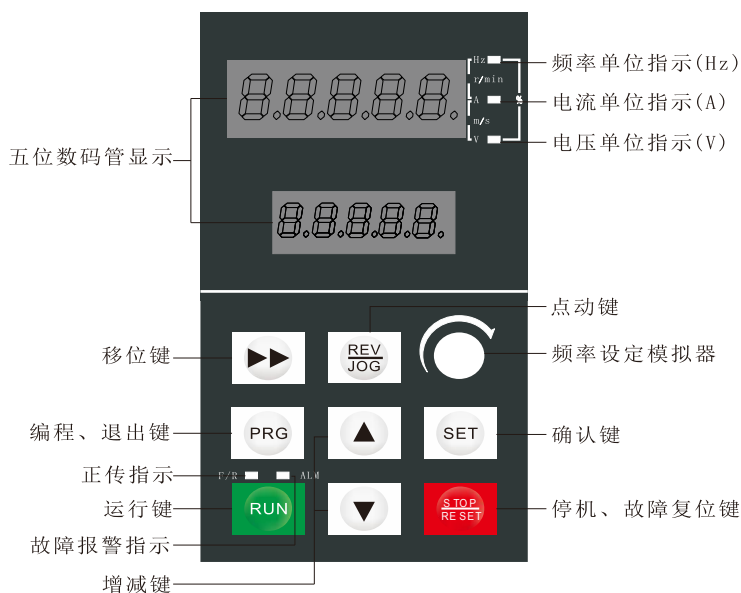
图4-2 操作面板示意图
