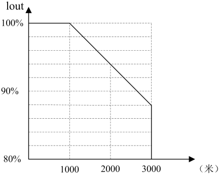
图 1-4 变频器额定输出电流与海拔高度降额使用图
