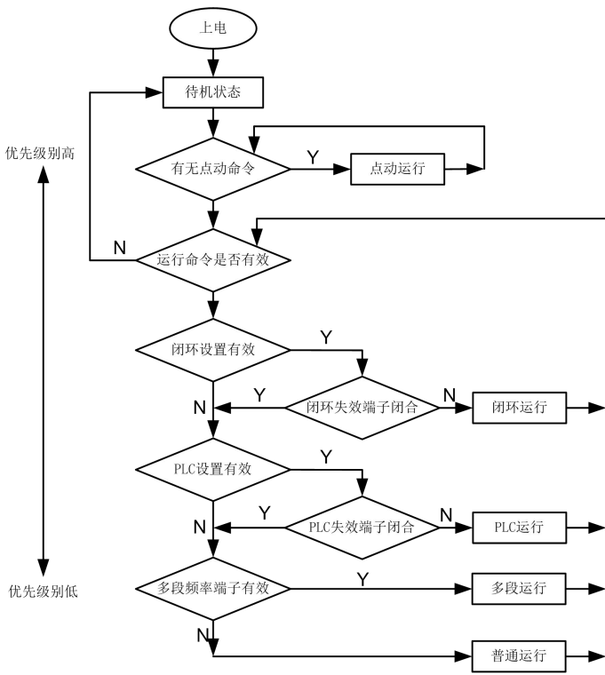
图 4-1 变频器运行状态的衍变逻辑
