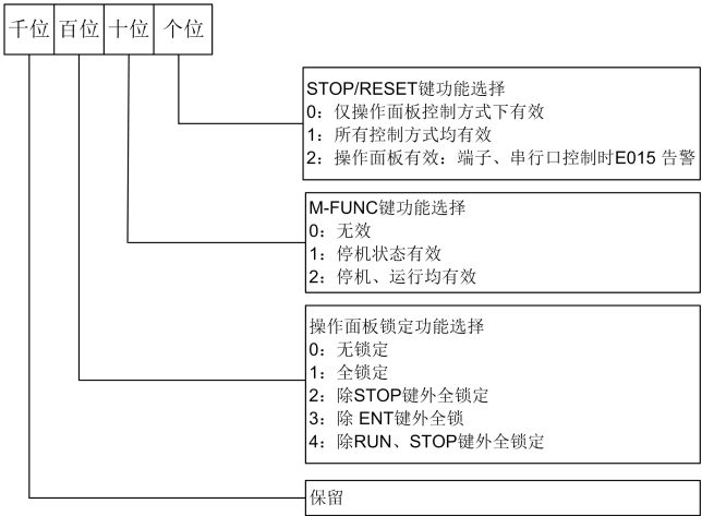
图6-70 操作面板按键功能及锁定选择设定
