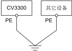
图3-13 接地示意图2
