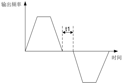
图 6-14 正反转死区时间
