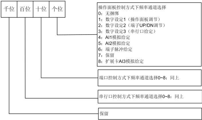
图 6-62 运行命令通道捆绑频率给定通道
