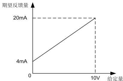
图6-38 给定量和期望反馈量
