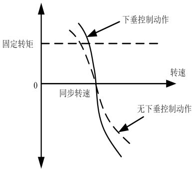
图6-60 下垂控制电机特性
