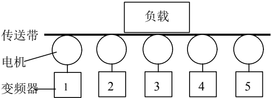
图6-59 下垂控制示意图
