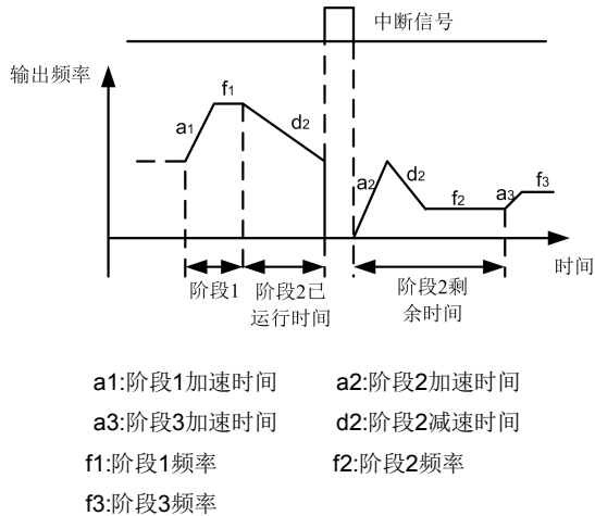
图6-50 PLC起动方式2
