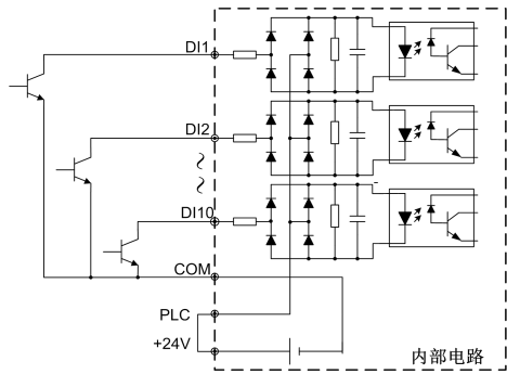
图 3-7 内部电源供电 NPN 图（OC）
