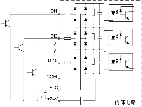
图 3-9 内部电源供电 PNP 图 (OE)
