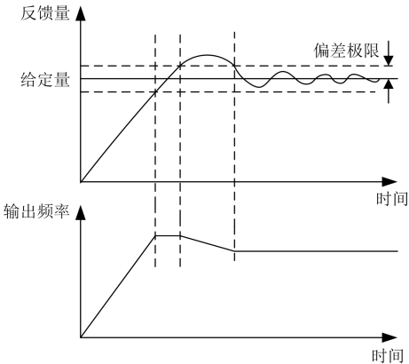
图6-42 偏差极限示意图
