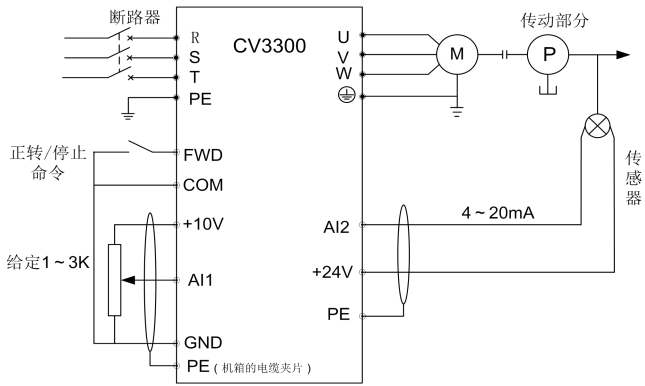
图6-35 内置PI模拟反馈控制系统示意图
