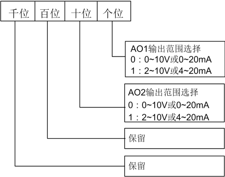
图6-33 模拟输出偏置设定
