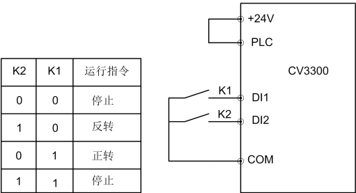
图6-25 两线式运转模式1
