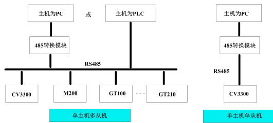
附图1 变频器组网方式示意图
