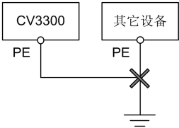
图3-14 接地示意图3
