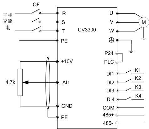
图6-64 三地控制硬件接线图
