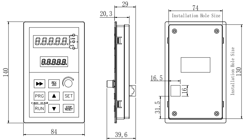
图 2-1 CV3300-RKD 键盘尺寸规格
