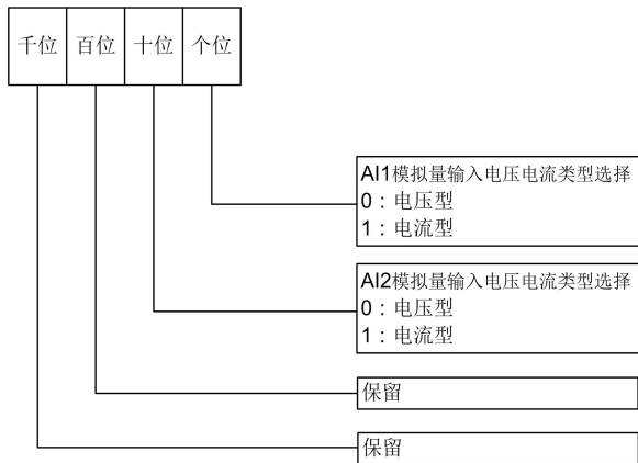
图 6-21 模拟量输入采样设置
