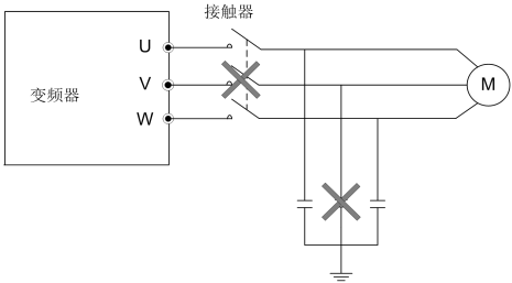
图 1-3 变频器输出端禁止使用电容器
