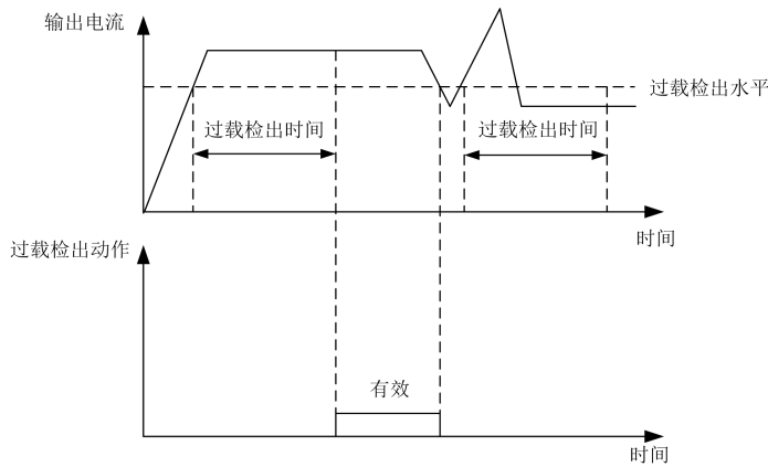
图6-54 过载预警检出功能示意图
