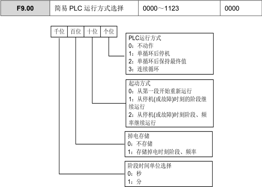
图6-45 简易PLC运行方式选择
