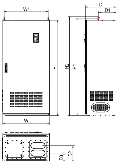
(d) 220KW~280KW 规格尺寸(柜机)
