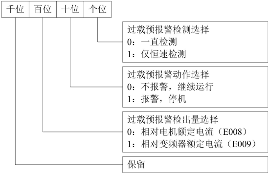
图6-53 过载检出设置设定
