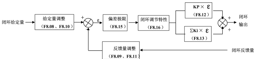
图6-37 PI原理框图
