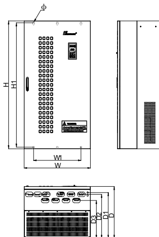
(b) 220KW~280KW 规格尺寸(壁挂)
