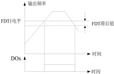
图6-29 频率水平检测示意图
