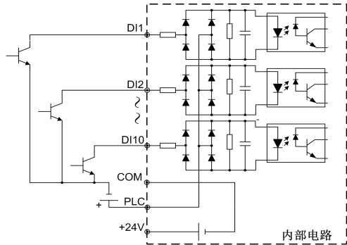
图 3-7 内部电源供电 NPN 图（OC）
