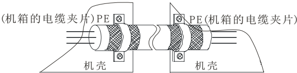
图3-16 正确的屏蔽接地方法
