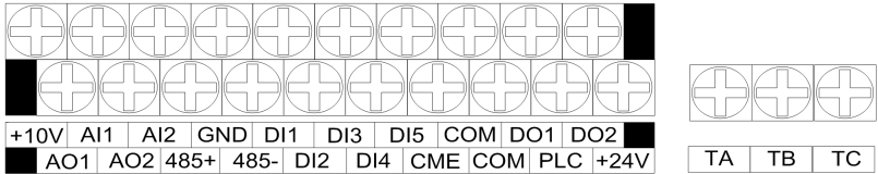
图 3-4 CV3300-4T0055G/4T0075P 及以上控制板端子排列顺序图
