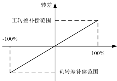
图6-58 自动转差补偿
