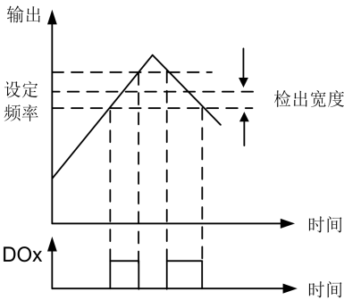
图6-30 频率到达信号输出示意图
