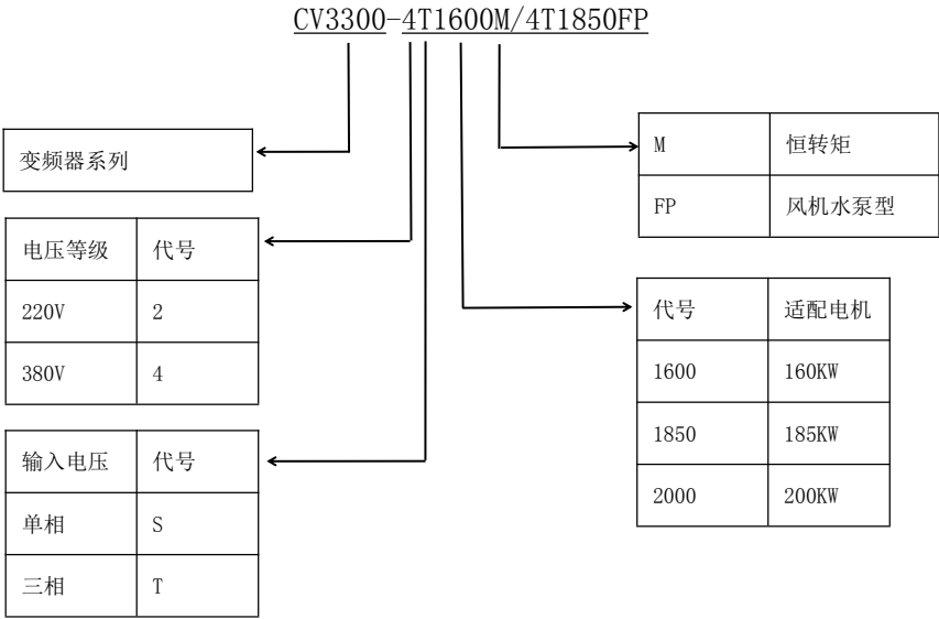
图 1-1 变频器型号说明
