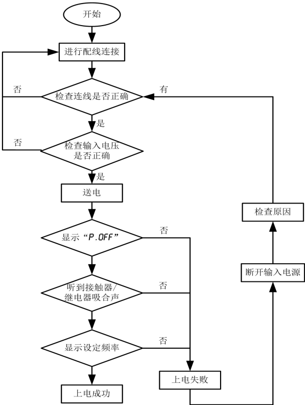
图 4-8 变频器初次上电操作流程
